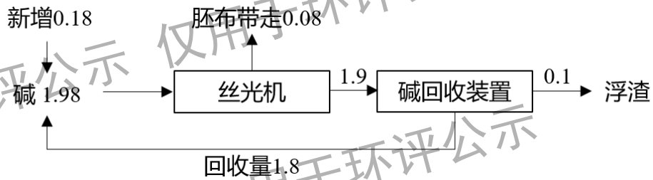
图 4.3-1 碱回收装置碱平衡图 (单位: t/d)
