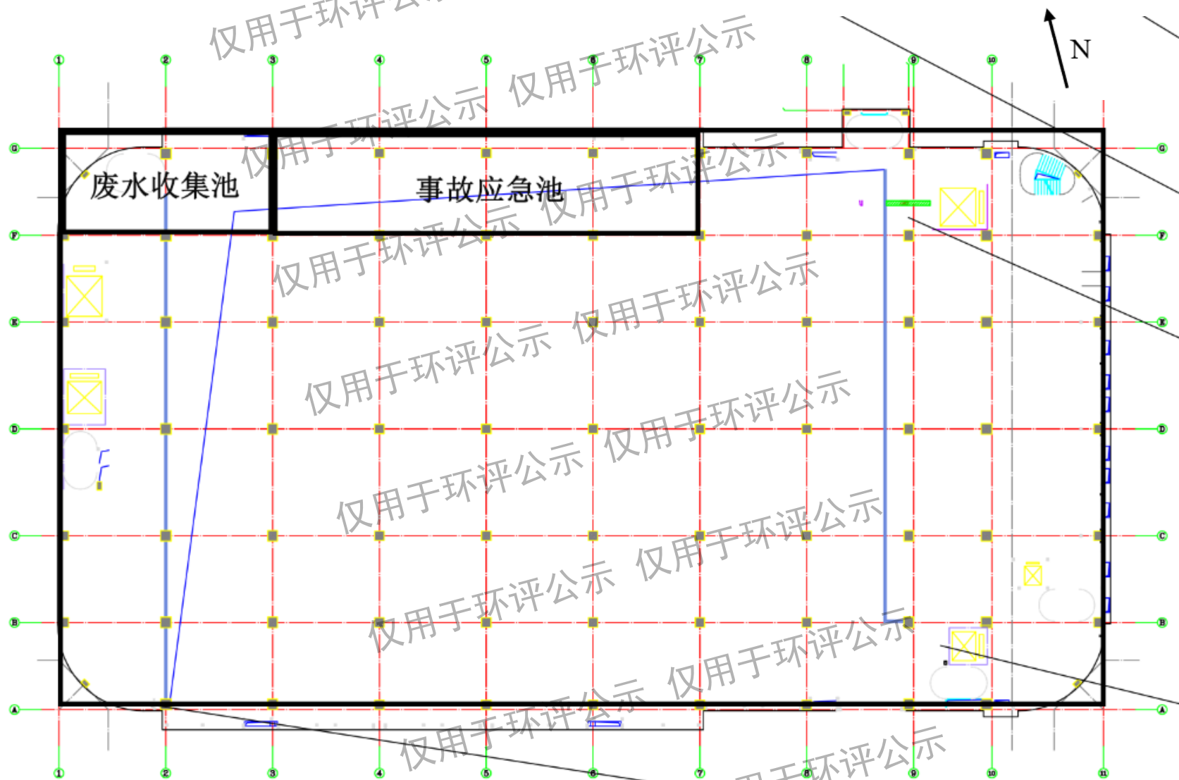
附图 6-7：厂房平面布置图（地下 2 层）
