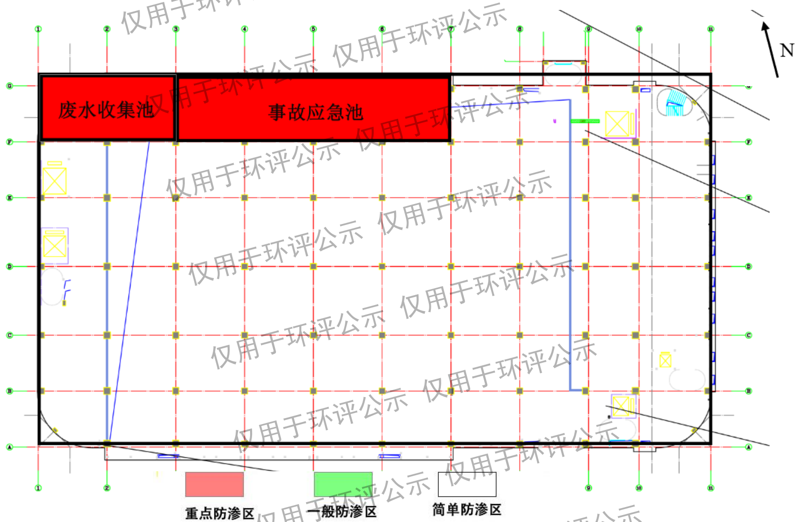
附图 9-2：地下水分区防治图（地下 2 层）
